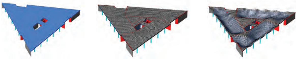
Abbildung 4.29: Übergabe an FEM Programm | Generieren FEM Netz | Anzeige der Verformungen (Quelle: Oltmanns &amp; Partner)
