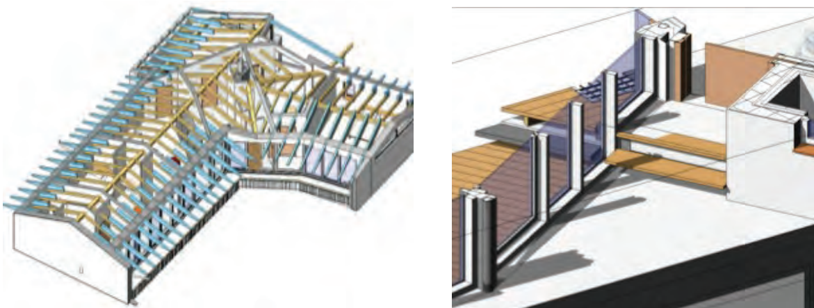
Abbildung 3.8: 3D Perspektive Gesamt- und Detaildarstellung (Quelle: Hobmaier, 3D ARCHITEKT)
