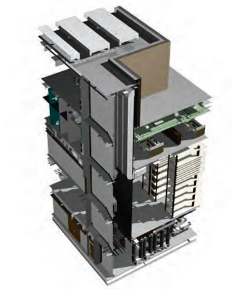
Abbildung 2.2: Querschnitt durch ein Bauwerksmodell Al Ain Hospital (Quelle: OBERMEYER Planen + Beraten)
