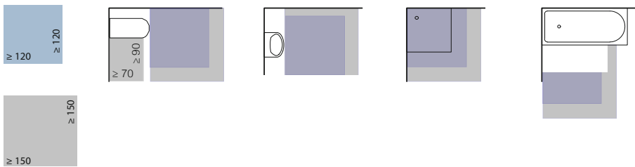
Abbildung 12: Bewegungsflächen vor Sanitärobjekten Anforderungen an Einrichtungen und Bewegungsflächen nach DIN 18040-2 (R) barrierefrei (blau) und rollstuhlgerecht (grau)
