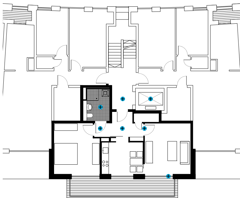
Grundriss Wohnung M 1:200
