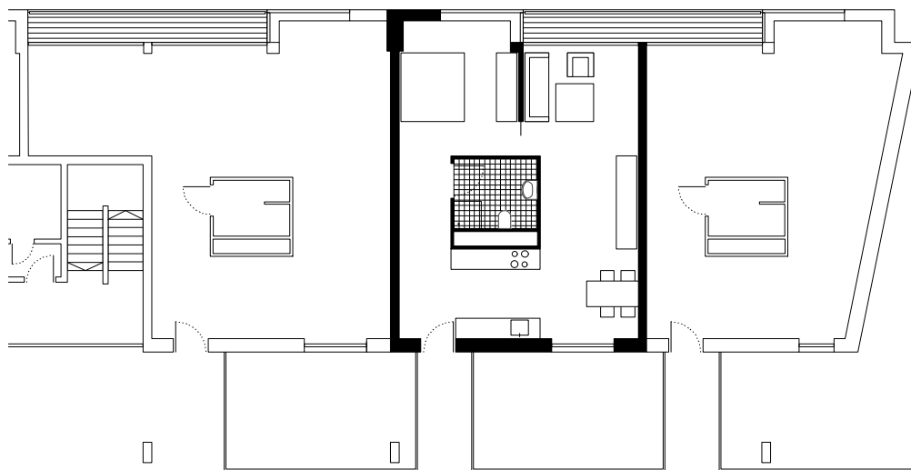
88 Grundriss Whg. M 1:200
