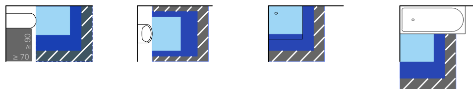
Abb. 6 Bewegungsflächen vor Sanitäröbekten nach DIN 18022:1989-11, DIN 18025:1992-12, bzw. DIN 18040:2011-09 Deutsche Planungsgrundlagen nach DIN 18022 (hellblau) und Anforderungen an Einrichtungen und Bewegungsflächen nach DIN 18025-2, bzw. 18040-2 barrierefrei (dunkelblau) und rollstuhlgerecht (schwarz)
