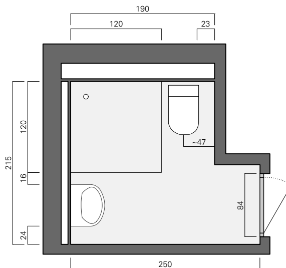
68 Grundriss Bad M 1:50
