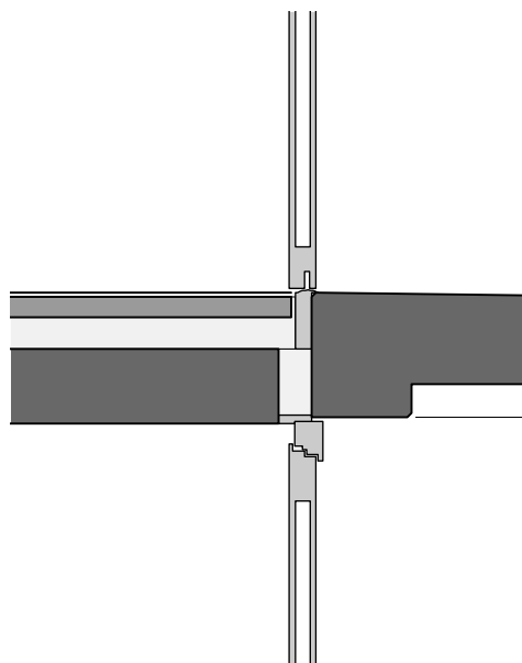
58 Detail Wohnungseingang 1:20
