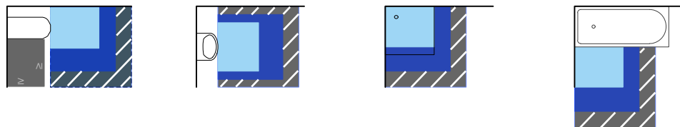
Abb. 24 Bewegungsflächen vor Sanitärobjekten nach DIN 18022:1989-11, DIN 18025:1992-12, bzw. DIN 18040:2011-09 Deutsche Planungsgrundlagen nach DIN 18022 (hellblau) und Anforderungen an Einrichtungen und Bewegungsflächen nach DIN 18025-2, bzw. 18040-2 barrierefrei (dunkelblau) und rollstuhlgerecht (schwarz)
