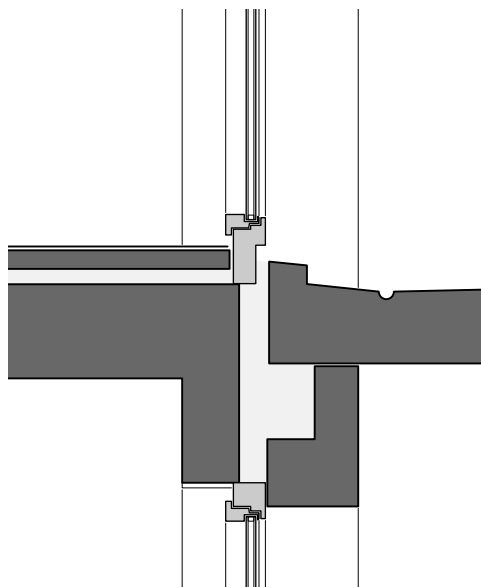
27 Detail Balkenschwelle M 1:20
